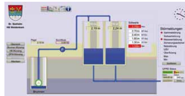
Erkennt Störungen und Wasserverlust: moderne Prozessleittechnik.
